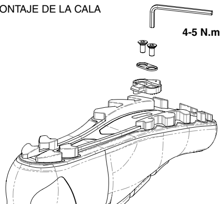
C / MONTAJE DE LA CALA
