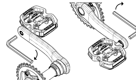
C / AJUSTE DEL PEDAL EN LA BIELA
