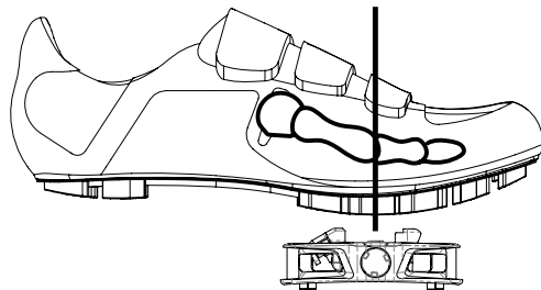
B / LONGITUDINAL POSITIONING
