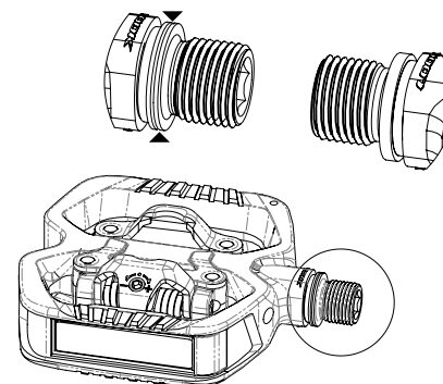
E / DIFERENCIACIÓN PEDAL DERECHO Y PEDAL IZQUIERDO
